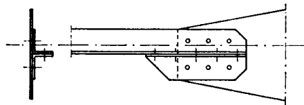
Figure 3.10: Lug angles
